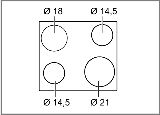
PKF6...17., PKF6..BB..
