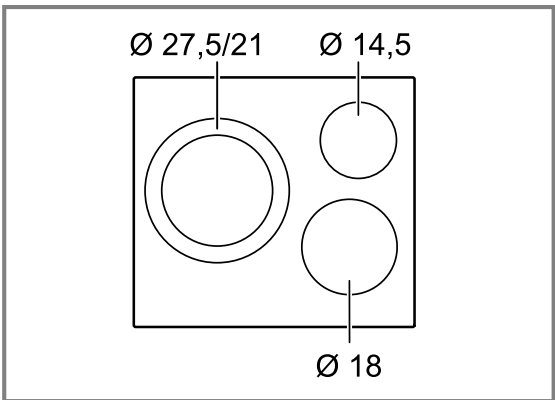
PKK6..B1..., PKK6..BB..
