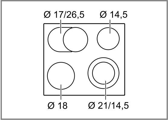
PKN6...17., PKN6..BB..
