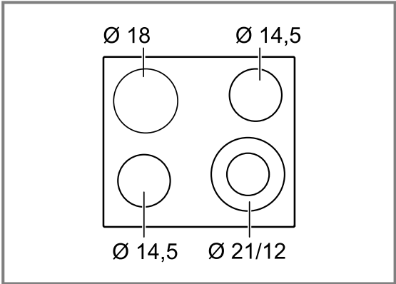
PKM6..B17., PKM6..BB..
