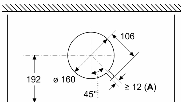
Mått i mm Vy ovanifrån
