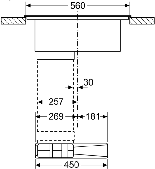
Mått i mm Frontvy
