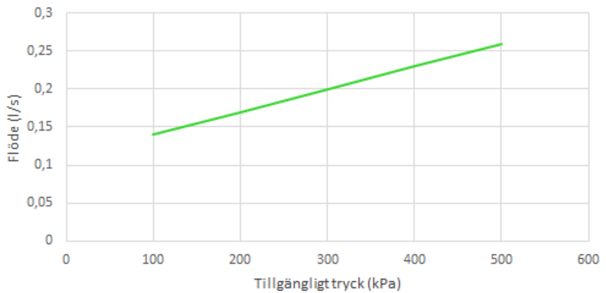
Tryckfallsdiagram BI071
